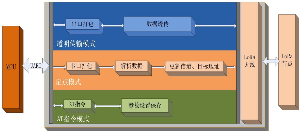
图 6 功能框图
