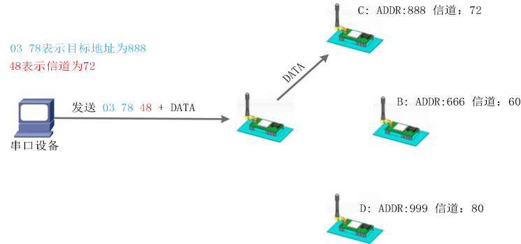
图 9 定点模式
