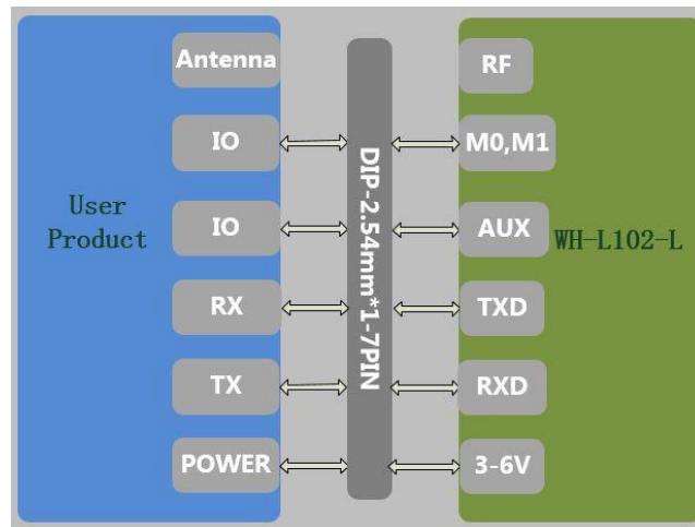
图 5 硬件连接
