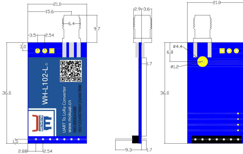
图 3 尺寸图
