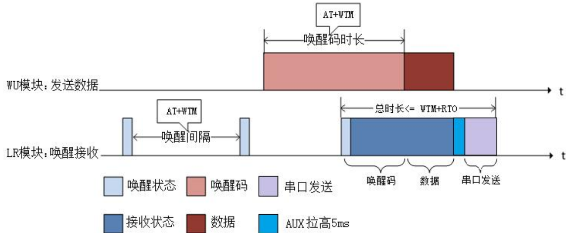
图 11 WU 和 LR 模式工作流程
