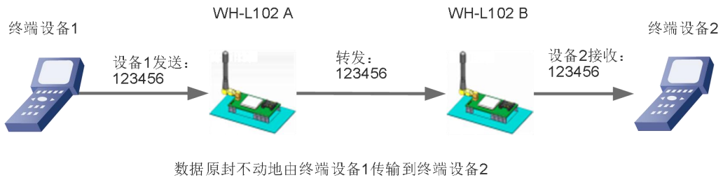
图 7 透传模式
