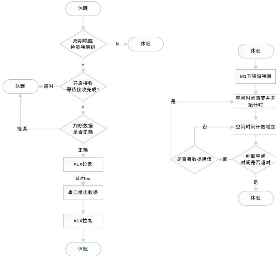
图 12 LR 模式工作流程
