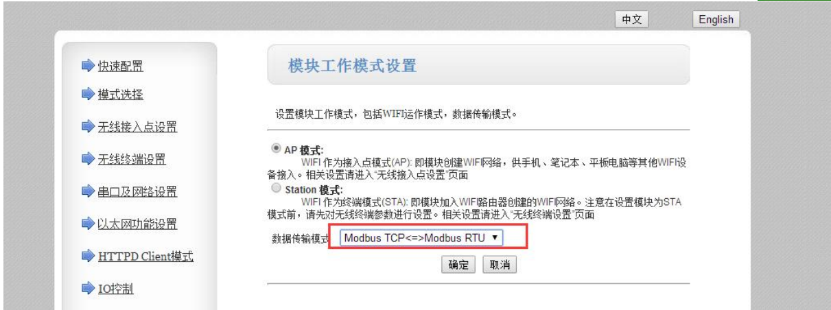
图 16 网页设置 Modbus RTU<=>Modbus TCP
