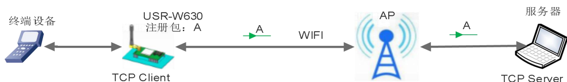
图 21 首次连接发送注册包框图
