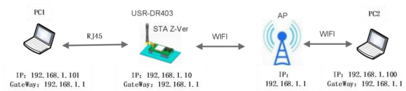
图 35 有线加无线组网应用（桥接）
