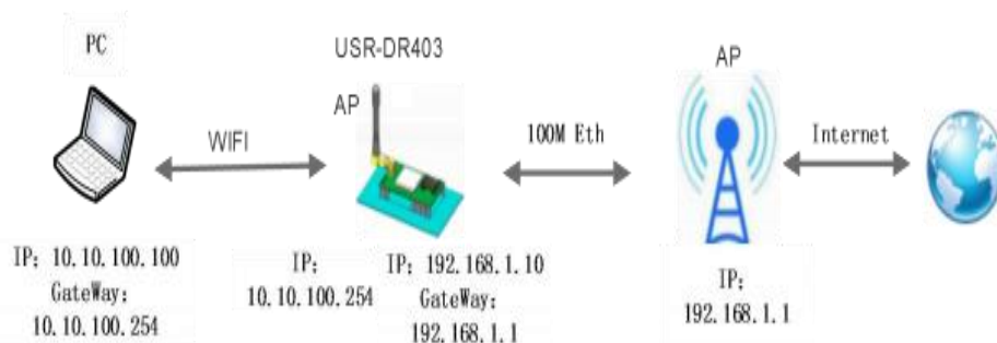
图 32 有线加无线的组网应用 (AP WAN)
