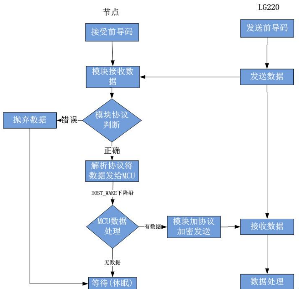
图 22 服务器主动下发简易流程
