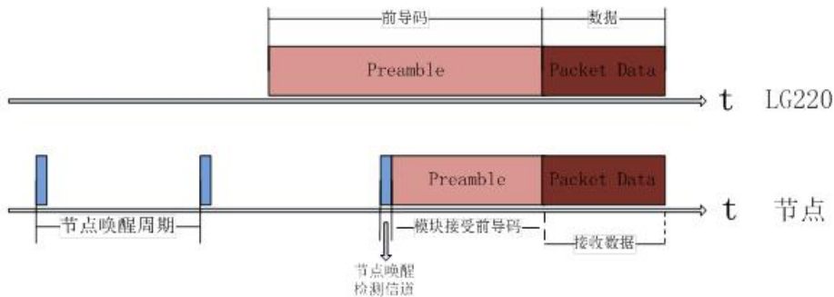
图 18 轮询唤醒模式时序
