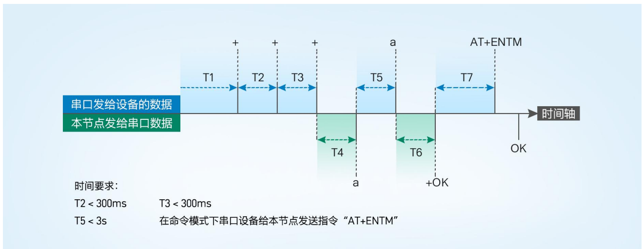
图 48 进入 AT 指令时序图
