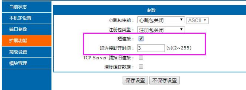
图 38. 短连接设置图示
