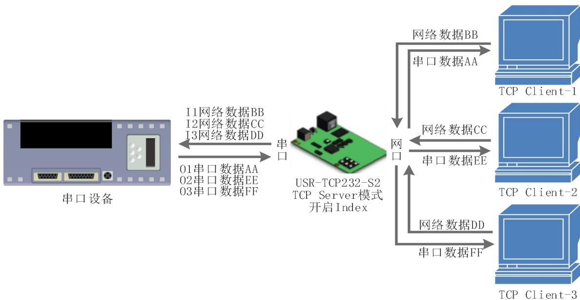
图 35. Index 功能示意图
