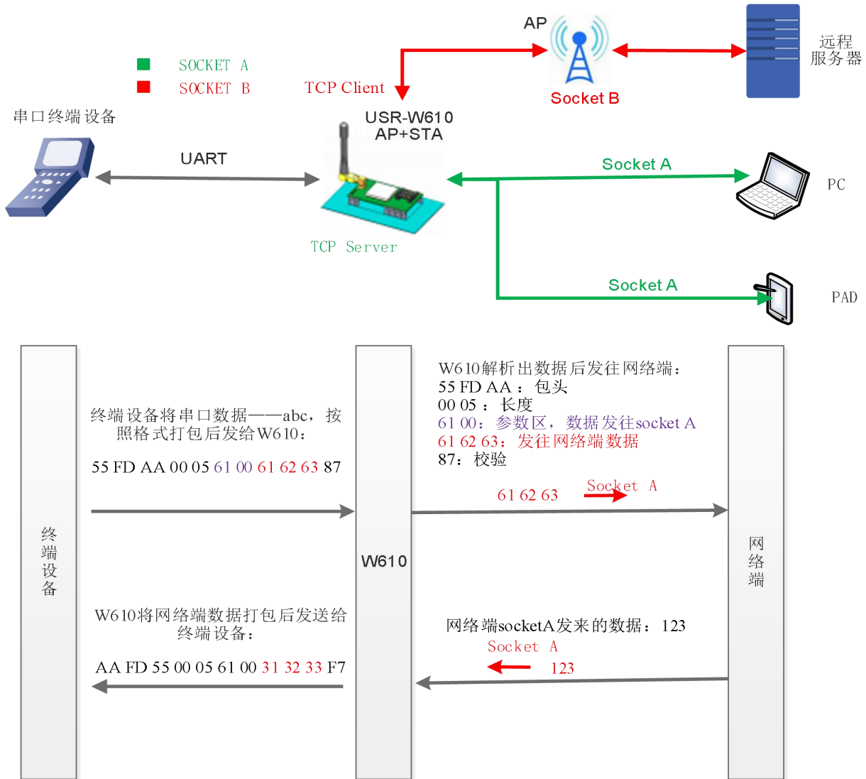
图 34 套接字分发框图
