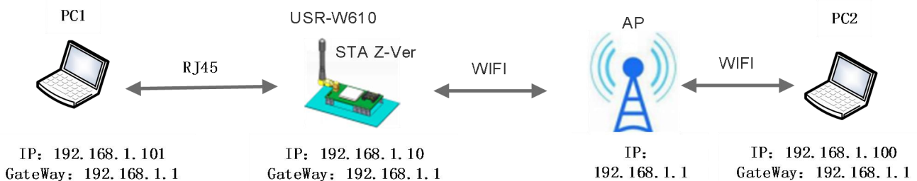
图 18 有线加无线组网应用（桥接）
