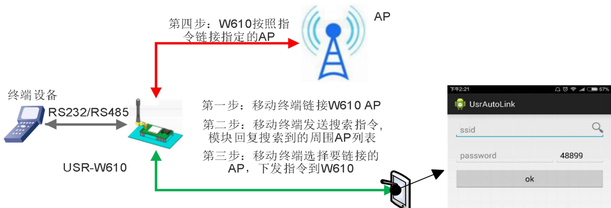
图 31 usr-link 框图
