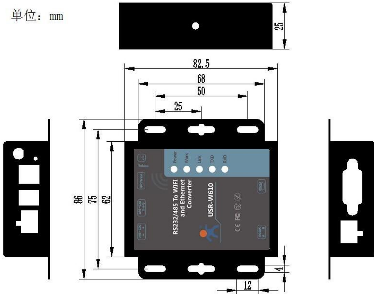
图 8 USR-W610 外观尺寸图
