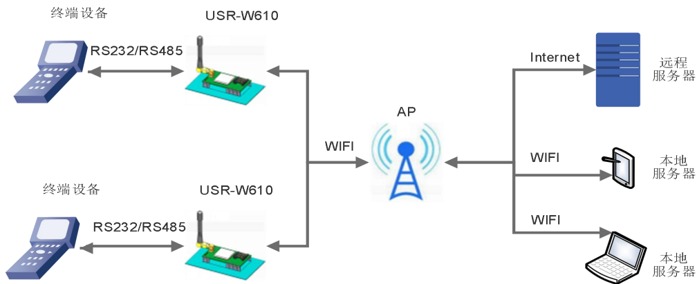
图 11 作为 STA 的应用场景
