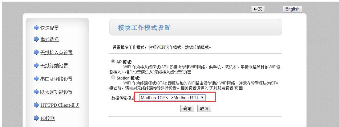
图 17 MODBUS TCP↔MODBUS RTU 模式选择
