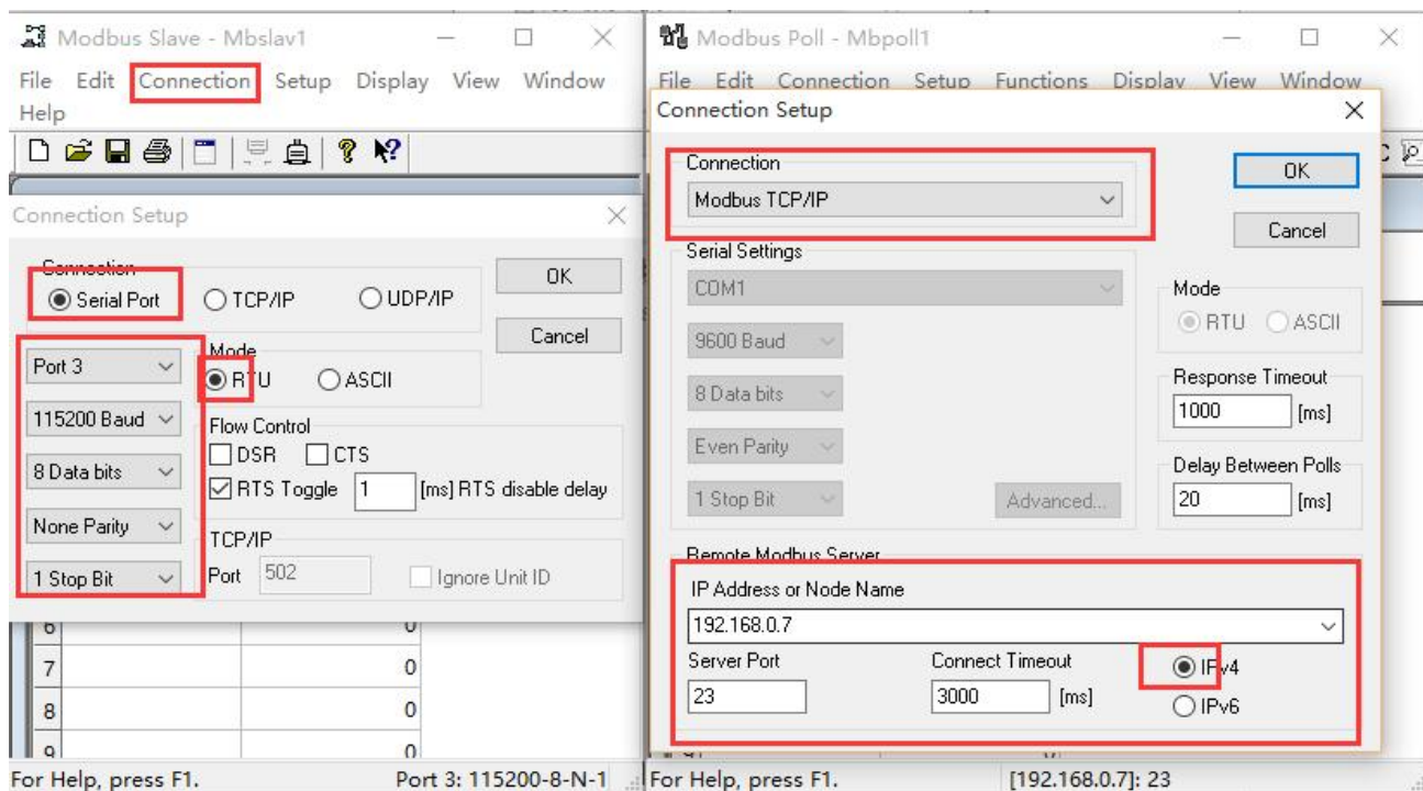
图 6. Modbus RTU 转 Modbus TCP 软件设置截图
