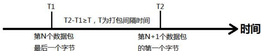
图 52. 时间触发模式
