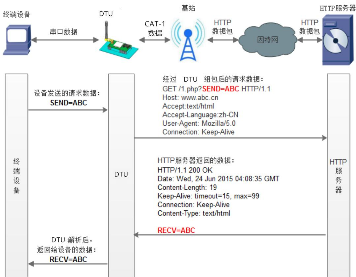
图 8. HTTPD Client 模式
