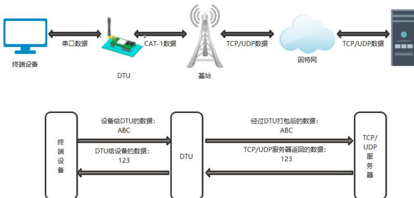
图 1. 网络透传模式
