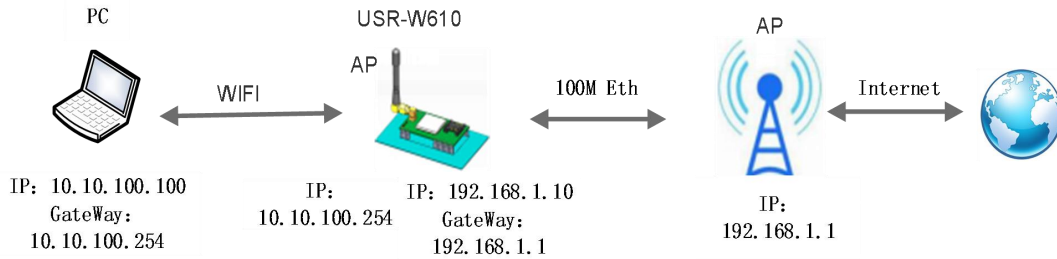
图 9 有线加无线的组网应用（AP WAN）
