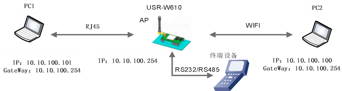
图 8 有线加无线的应用场景（AP LAN）
