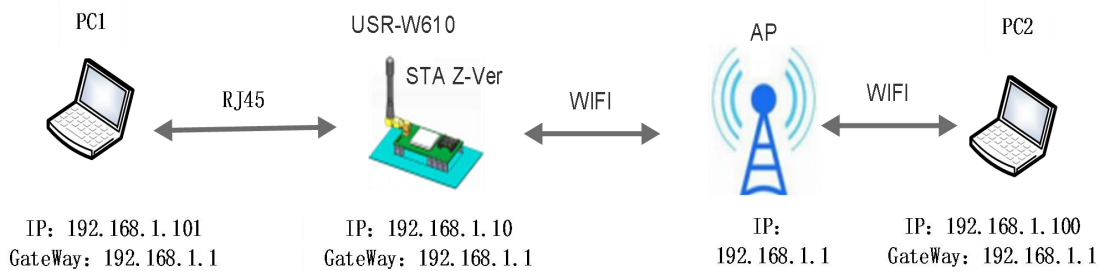
图 12 有线加无线组网应用（桥接）
