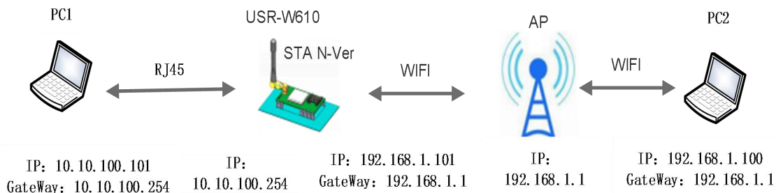
图 10 有线加无线组网应用（路由）
