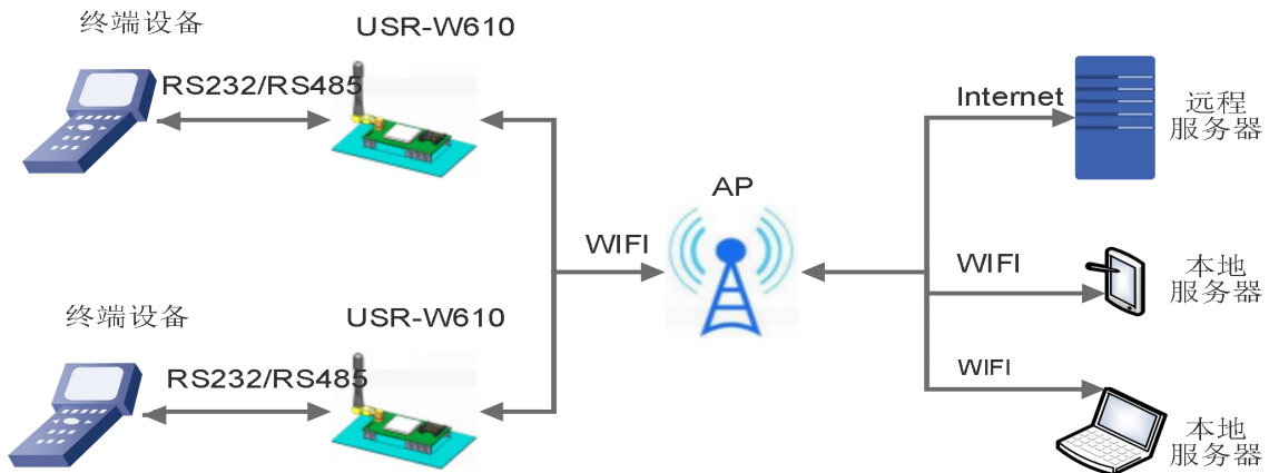
图 4 无线组网应用 (STA)
