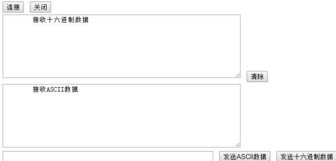
图 38 WebSocket 页面
