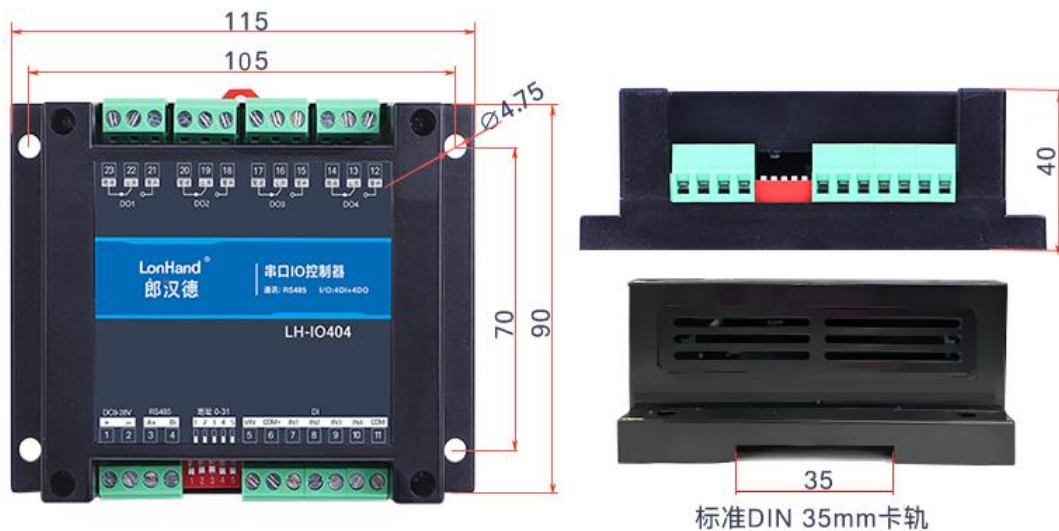
LH-IO404 尺寸: 115*90*40 单位: mm
